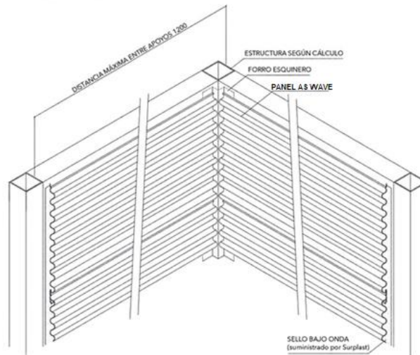
DETALLE ESQUINA
