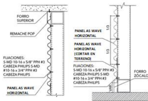
DETALLE REMATE SUPERIOR E INFERIOR
